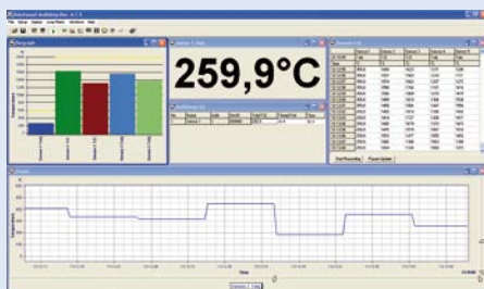
Courbes de valeurs mesurées par plusieurs capteurs placés en réseau, avec représentation de valeurs alarmes pour la détection du dépassement des valeurs seuils.
