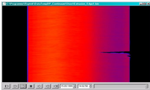
Fig. 27: Image thermique d'un film plastique avec détection d'un défaut sur son bord droit.
