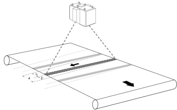
Fig. 28: Principe de mesure d'un scanner en ligne
