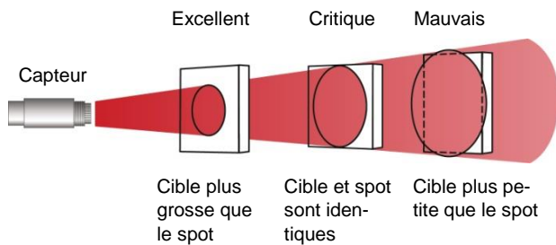
Fig. 17: La cible doit totalement remplir le spot de mesure. Dans le cas contraire la mesure sera affectée (exception : Pyromètre bichromatique)
