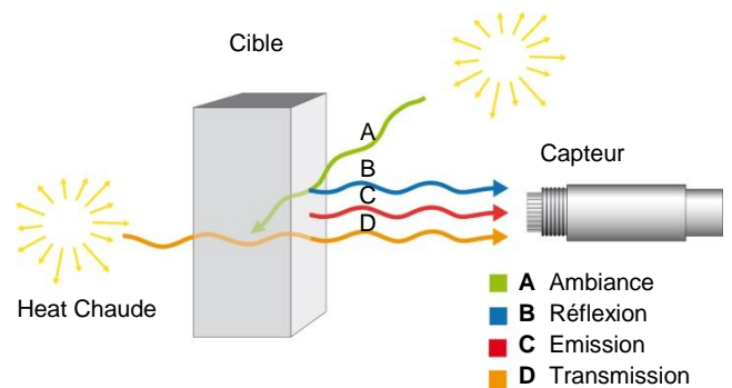
Fig. 6: En plus de l'énergie émise par la cible, le capteur peut recevoir de l'énergie réfléchiée et de l'énergie transmise.
