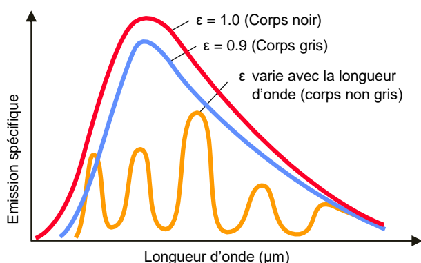
Fig. 7: Emission spécifique à différentes longueurs d'onde
