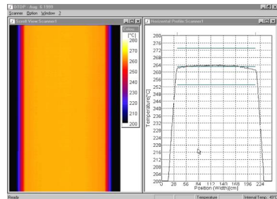
Fig. 29: Copie d'un écran de scanner en ligne mesurant un film en mouvement. Image thermique à gauche et profil à droite.
