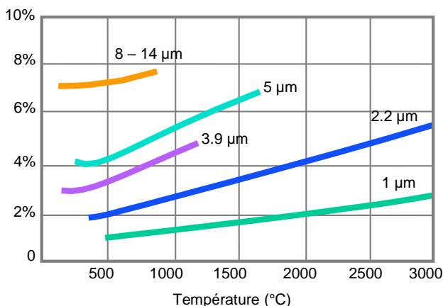
Fig. 8: Erreur de mesure causée par un écart de 10% entre la valeur vraie et la valeur ajustée de l'émissivité pour différentes longueurs d'ondes et différentes températures.
