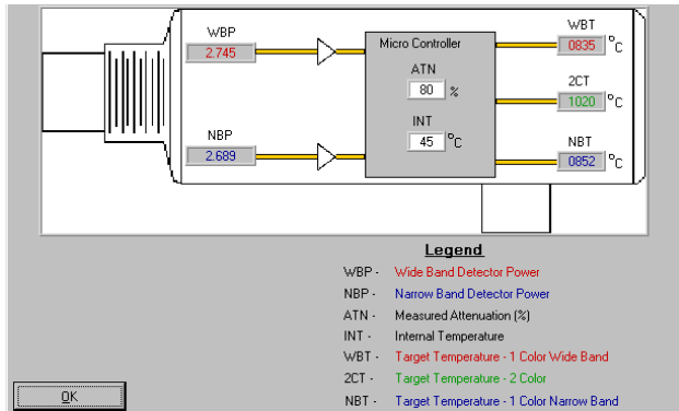
Fig. 26: Informations données par le logiciel d'un pyromètre bichromatique. Ex. Temp. mono voie 1 (WBP), Temp. mono voie 2 (NBP) et Temp. bi. (2CT). L'atténuation (ATN) est aussi calculée et affichée.
