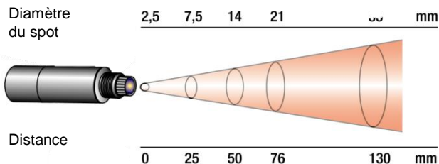
Fig. 18: Caractéristique optique d'un capteur IR. A une distance de mesure de 130 mm, le diamètre du spot de mesure est de 33 mm. Sa résolution optique est 130/33 = 4/1
