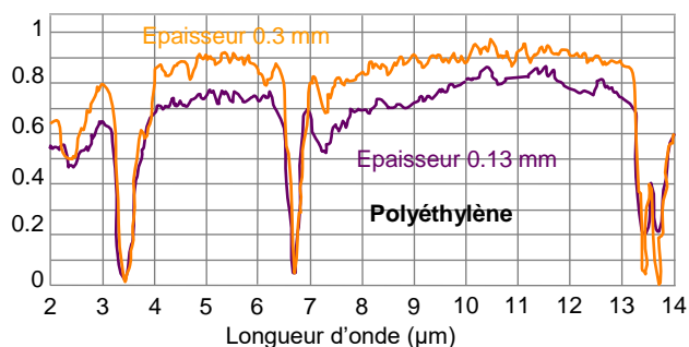
Fig. 10: Transmission spectrale des films plastique. Quelque soit son épaisseur, un film polyéthylène est opaque à 3,43 µm.
