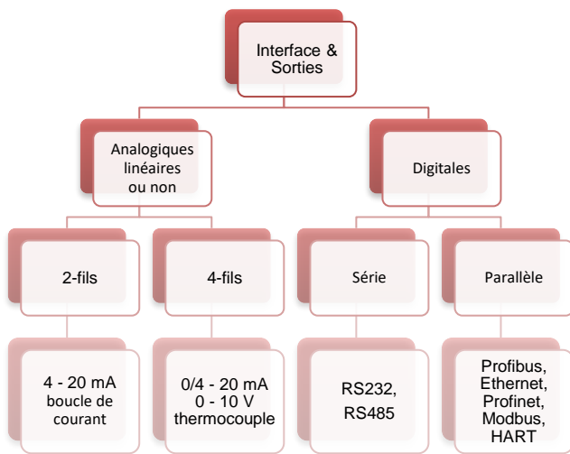
Fig. 24: Exemples d'interfaces disponibles sur les capteurs IR
