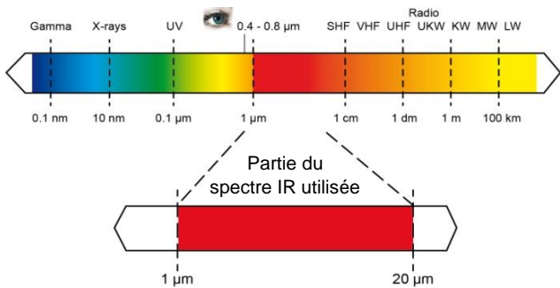
Fig. 4: Le spectre électromagnétique. Seule la partie allant de 1 à 20 µm est utilisée en mesure IR.
