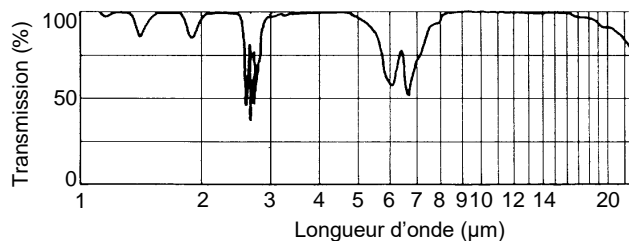
Fig. 14: Transmission spectrale d'une couche d'air de 1 m d'épaisseur à 32°C et 75% d'humidité relative. /3/
