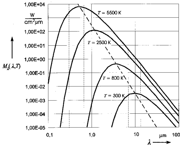
Fig. 5: Emission d'un corps noir en fonction de la température. /3/
