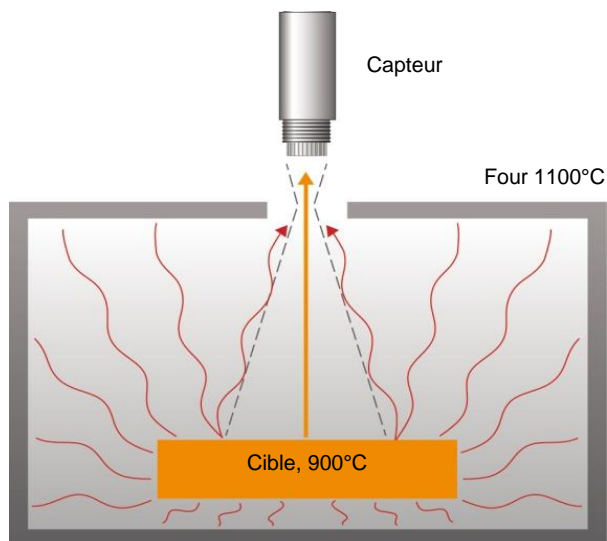
Fig. 15: La compensation de température ambiante est importante lorsque la cible est plus froide que son environnement.
