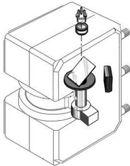
Fig. 30: Principe de fonctionnement d'un ensemble opto-mécanique avec miroir tournant.
