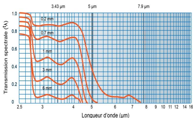
Fig. 12: La transmission spectrale du verre dépend de son épaisseur
